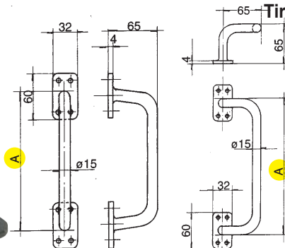
Art. 482 Tipo diritto Type droit Right model Tipo recto
