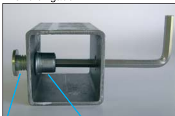
distanziatore 878 boccola filettata 878/A
