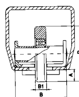
Art. 2110/M Art. 2110/P ruota di sostegno Roue de support Support wheel Rueda soporte final
