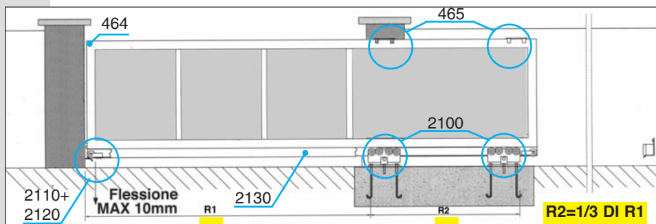
Art. 2110/M Art. 2110/P ruota di sostegno Roue de support Support wheel Rueda soporte final
