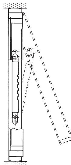
Art. 340 per apertura a sporgere pour ouverture vers extérieur for outside going window
