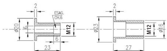
distanziatore 878 boccola filettata 878/A
