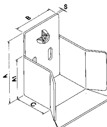
Art. 2120/M Art. 2120/P Incontro Butée Staple Encuentro
